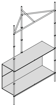
ELLE 1002 single module with 2 shelves modulo singolo con 2 ripiani
