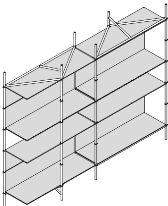
ELLE 100C1 + 1005 system with 2 modules with 7 shelves sistema con 2 moduli e 7 ripiani
