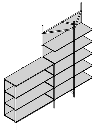
ELLE 100C3 + 1005 system with 2 modules with 9 shelves sistema con 2 moduli e 9 ripiani
